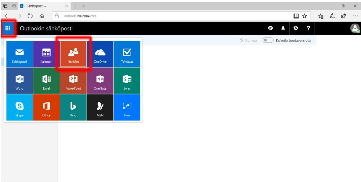
Kuva 1 Sähköpostin kirjautumisnäkyvä
