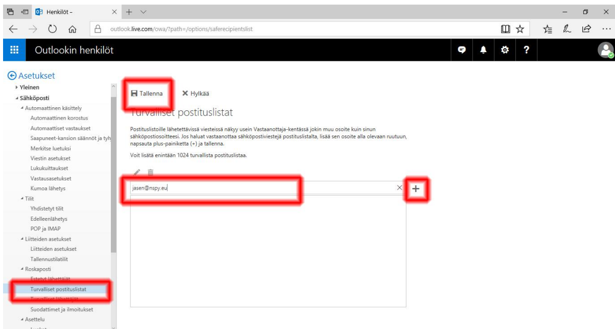
Kuva 4 Turvalliset postituslistat
